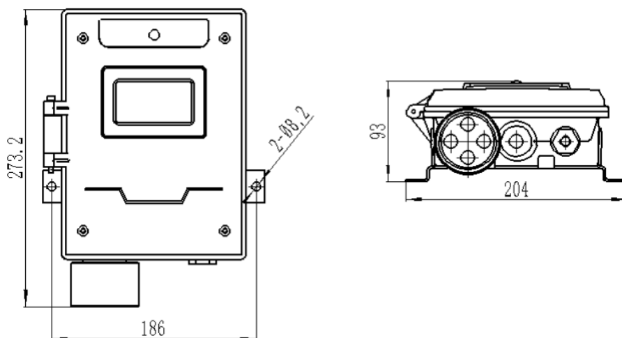
Рисунок 3.1 Габариты
