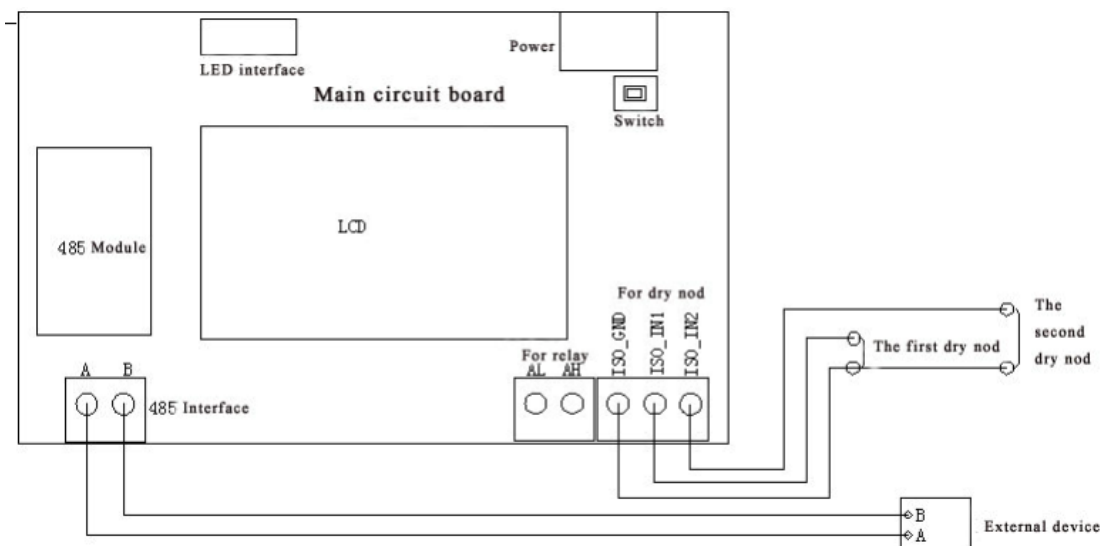
Рисунок 3.2 Схема подключения
