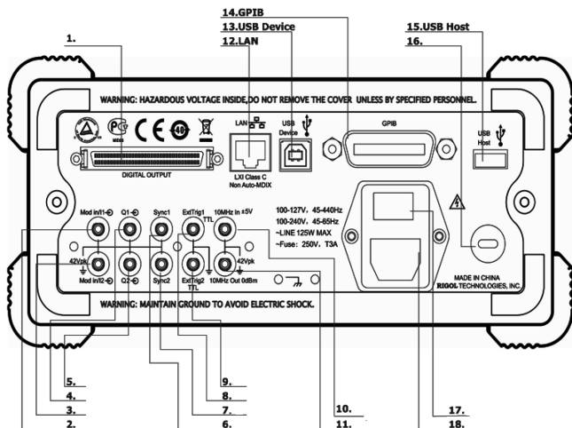
Задняя панель двухканального генератора
