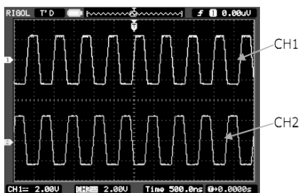
Вид до нажатия кнопки Restore
