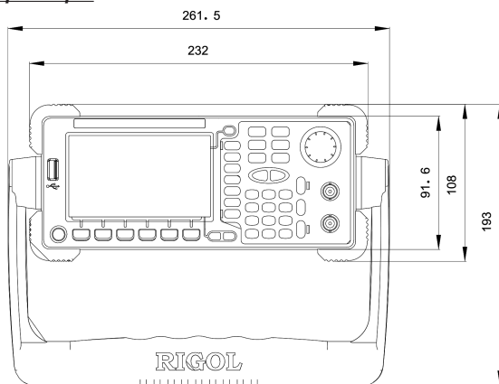
Вид спереди, единица измерения: мм
