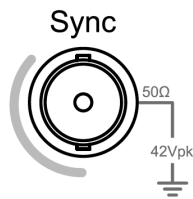
Коннектор [Sync] одноканальной модели
