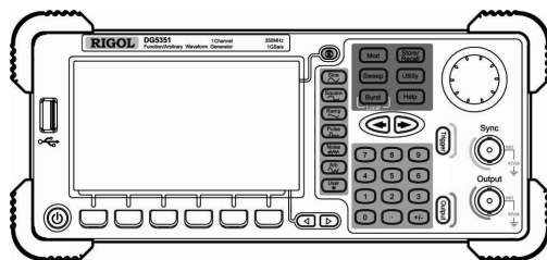
Передняя панель одноканального генератора
