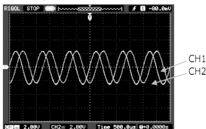
До выравнивания фаз
