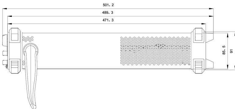
Вид сбоку, единица измерения: мм
