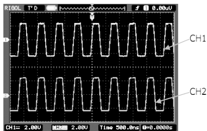
Вид после нажатия кнопки Restore
