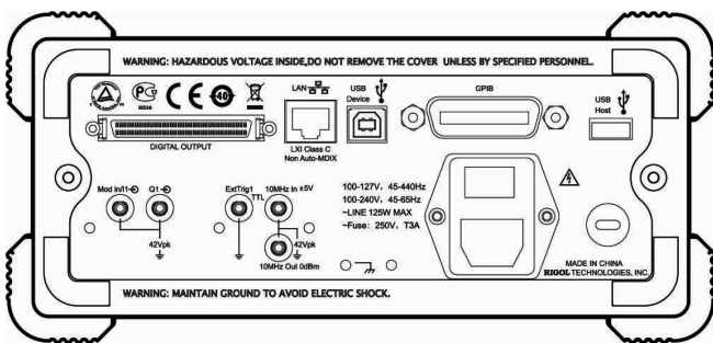
Задняя панель одноканального генератора
