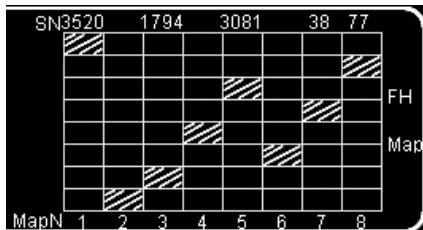
Диаграмма перескока по частоте «Chess»
