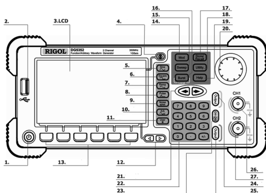
Передняя панель двухканального генератора
