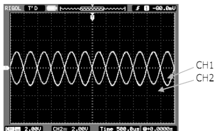
После выравнивания фаз
