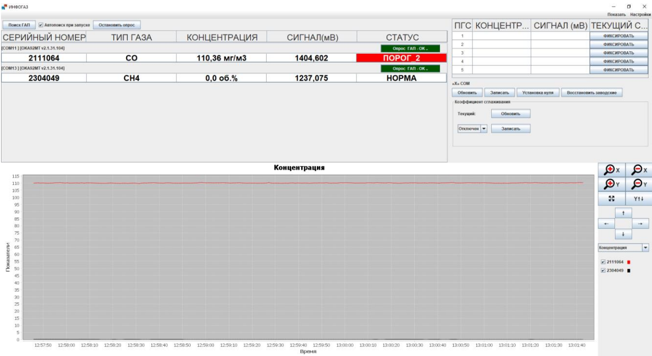
Рис. Б6 Основное окно в режиме калибровки
