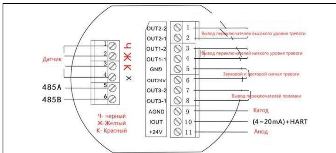
Рис.8 : Соединительные клеммы
