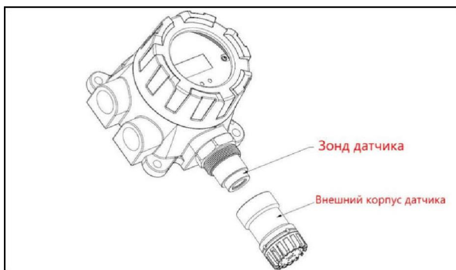
Рис. 22 : Замена датчика
